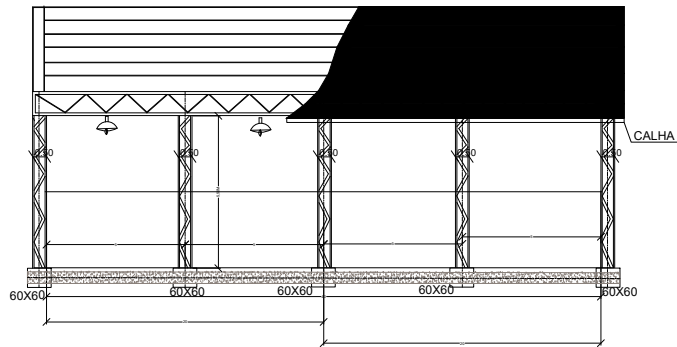
Planta -Corte BB Esc. 1/50
