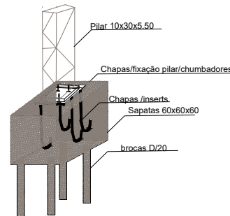
Detalh. Fixação Pilares /Chumbadores Sem/Esc.
