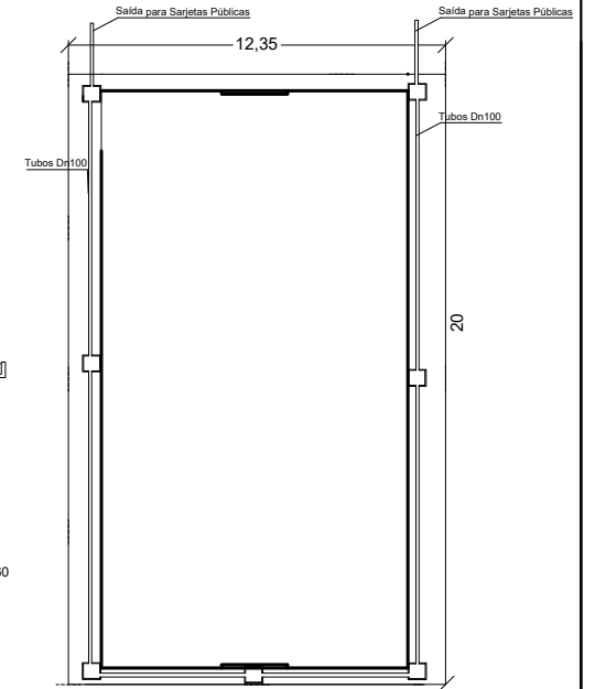
Planta-Localização caixa de passagem /Dreng Esc. 1/50 caixas conforme especificadas em planilha
